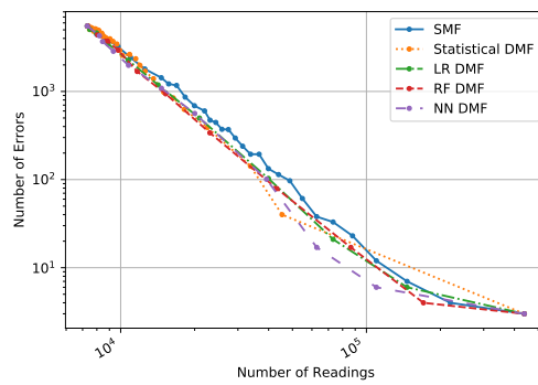
(d) Results for temperature dataset, \Delta_{max} = 1.5^{\circ}\text{C}
